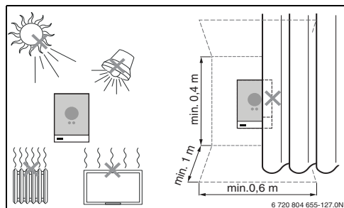
Afb. 4 Montageplaats thermostaat
