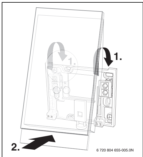
Afb. 6 Monteren thermostaat
