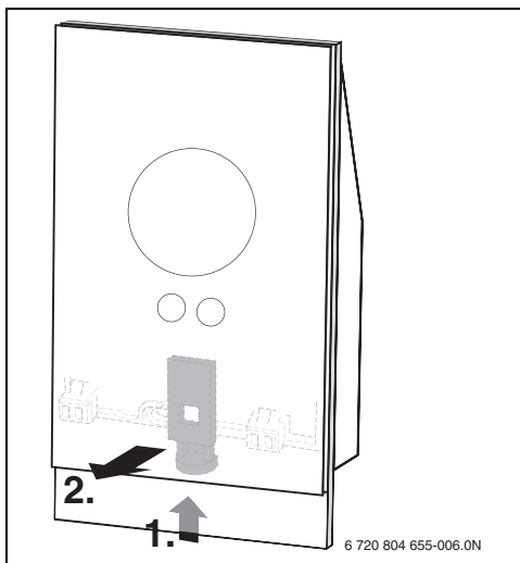
Afb. 7 Demontage thermostaat
