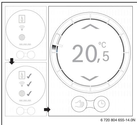
Afb. 10 Geslaagde installatie
