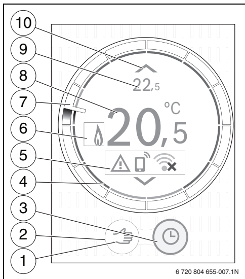
Afb. 2 Overzicht touchscreen
