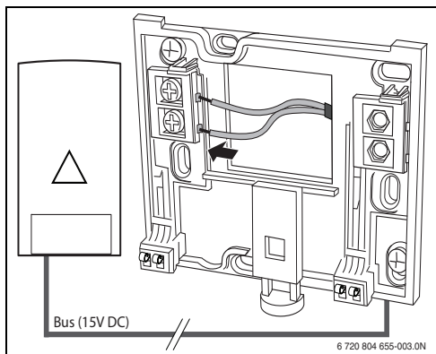
Afb. 5 Aansluiten grondplaat
