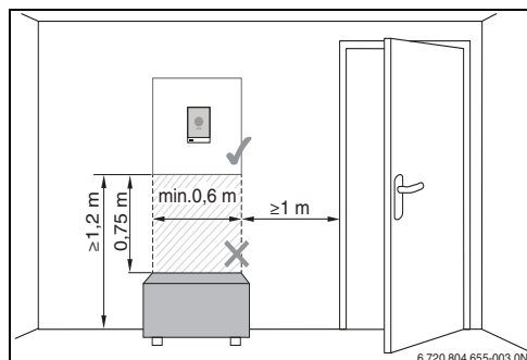
Afb. 3 Montageplaats thermostaat - vrije ruimte
