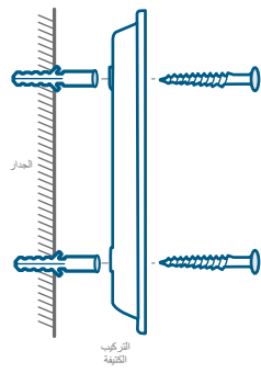
بدون إسفين متصاعد بمقدار 15 درجة
