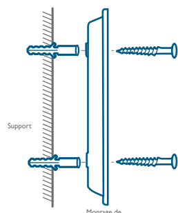
Sans cale de montage 15°
