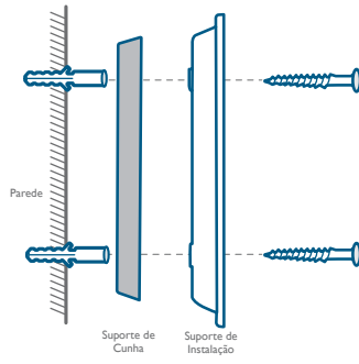
Com a cunha de instalação de 15°
